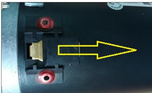
Figuur 5b & c: Koolborstels inspecteren reinigen
