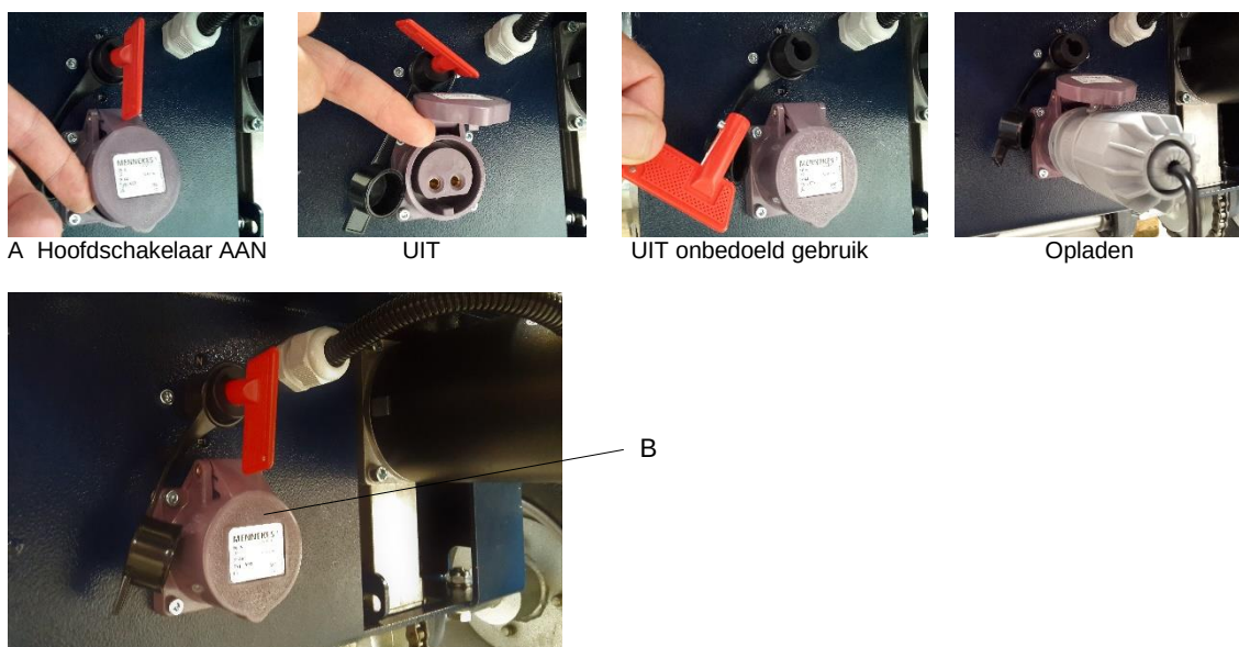
Figuur 3: Onderwagen EasyTrack
