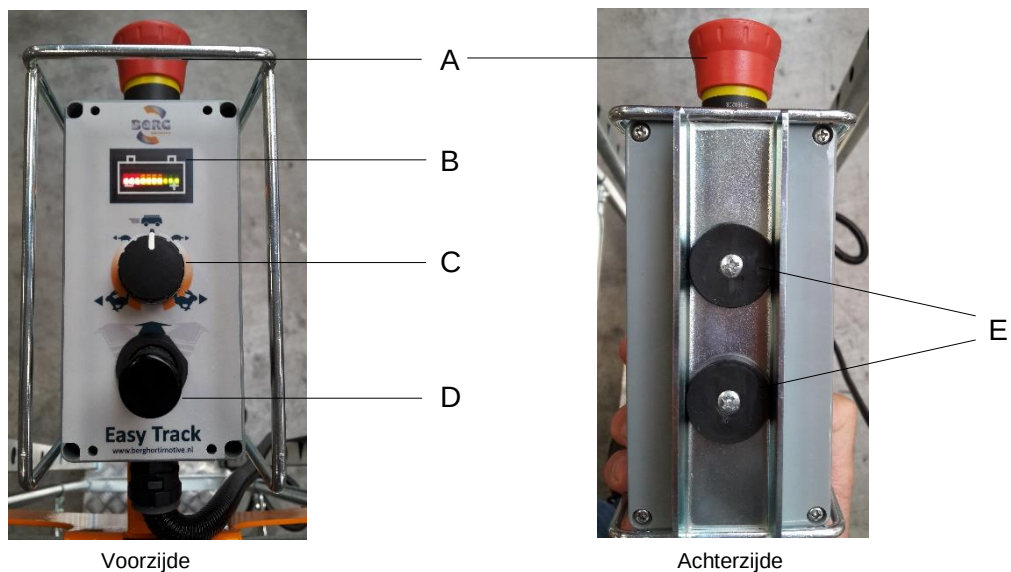
Figuur 2: Bediening EasyTrack
