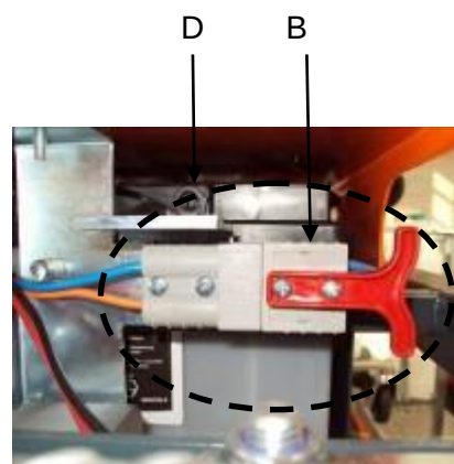
Figuur 4. massaslot
