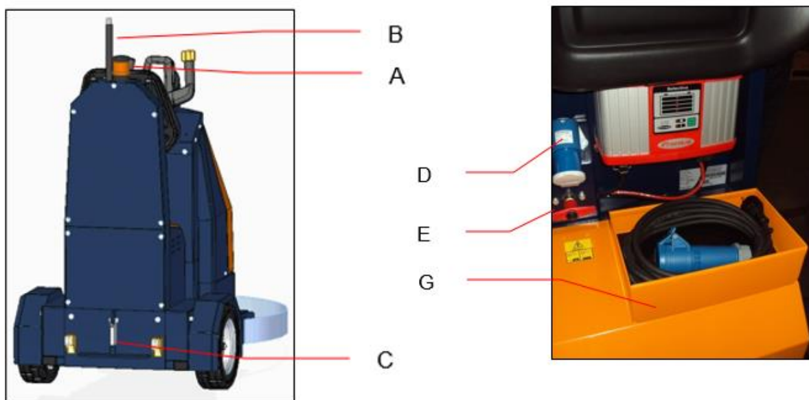
図 5: BeTrac 1 AGV のその他コンポーネント
