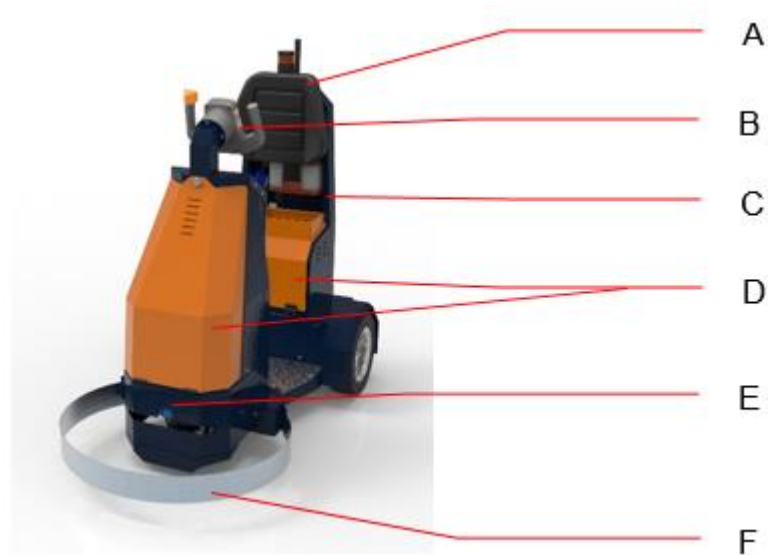
図 1: BeTrac 1 AGV の主なコンポーネント
