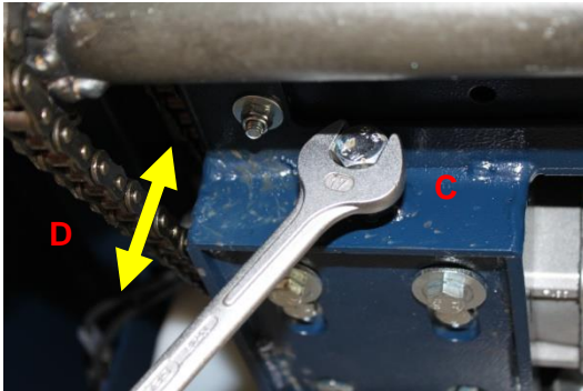
Figuur 9.5 A-B-C; Spannen van de ketting
