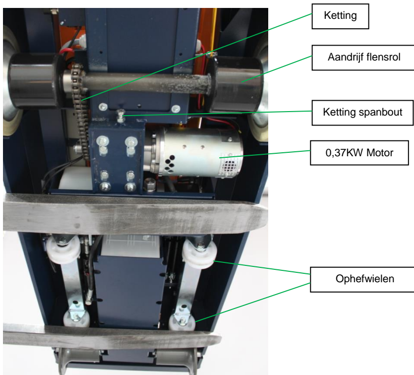
Figuur 5.2; Benaming van de onderdelen aan de onderzijde van de Benomic STAR 260
