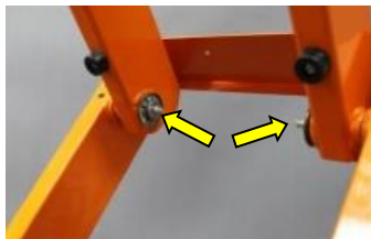
Figuur 9.2; Positie van de smeernippels voor de schaarassen
