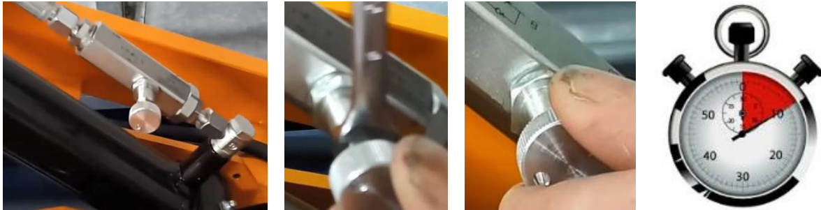
Figuur 9.6; Daalsnelheid schaarplateau afstellen
