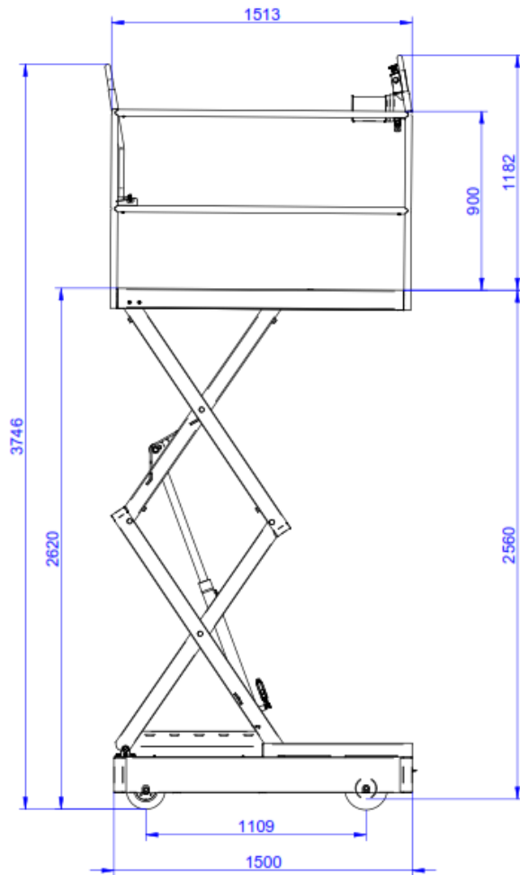
Fig. 2.1; Maximale afmetingen 2-schaar in mm
