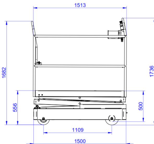
Fig. 2.2; Minimale afmetingen 2-schaar in mm
