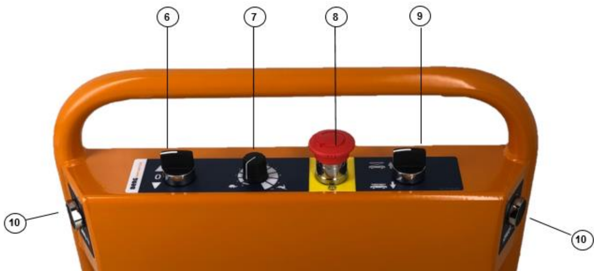
Fig. 8.3; Bedieningsconsole
