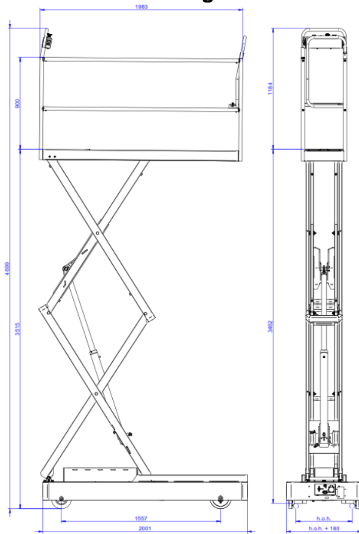
Fig. 2.3; Maximale afmetingen 2-schaar in mm
