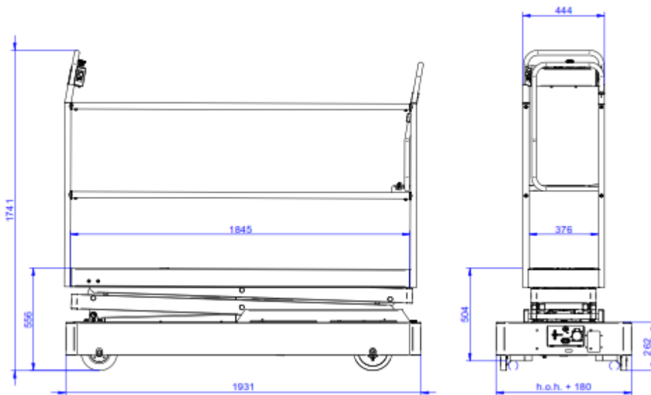
Fig. 2.2; Minimale afmetingen 2-schaar in mm
