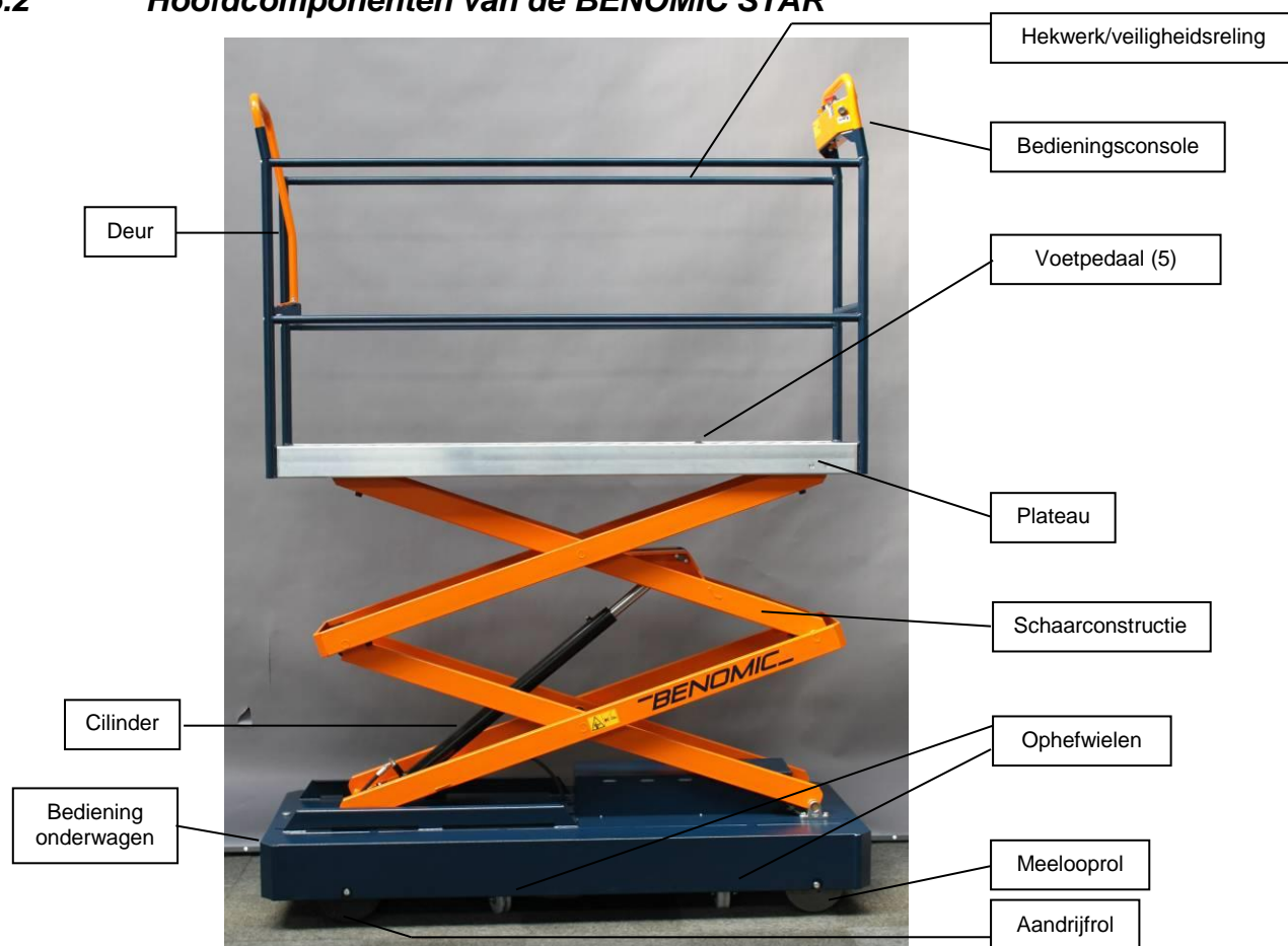
Figuur 5.1; Benaming van de onderdelen aan de bovenzijde van de BENOMIC STAR
