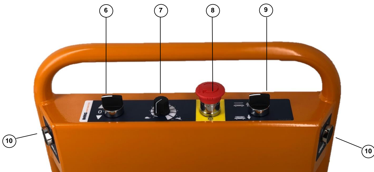
Fig. 8.3; Bedieningsconsole
