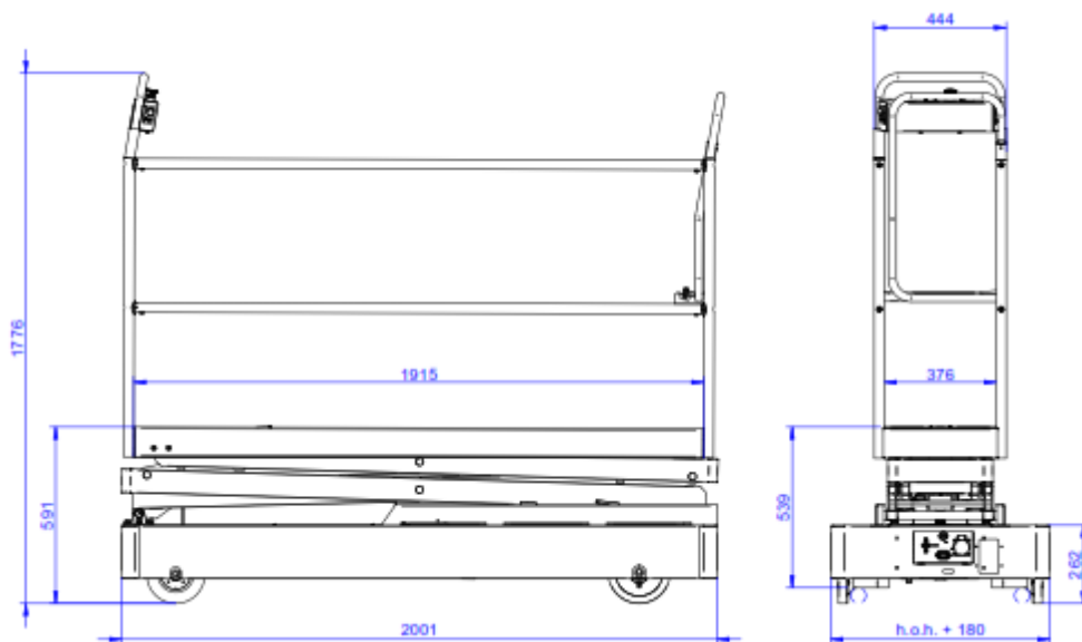
Fig. 2.4; Minimale afmetingen 2-schaar in mm
