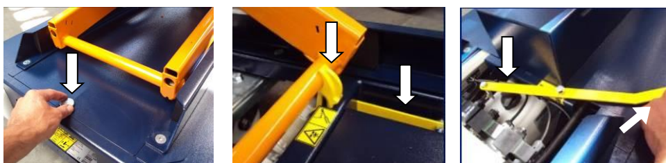
Fig. 8.4; Links: bout losdraaien en kap wegnemen. Midden; veiligheidsbal omhoog & hendel uitnemen. Rechts; Bout in gat en bout tegen pen van het nooddaalventiel drukken!!
