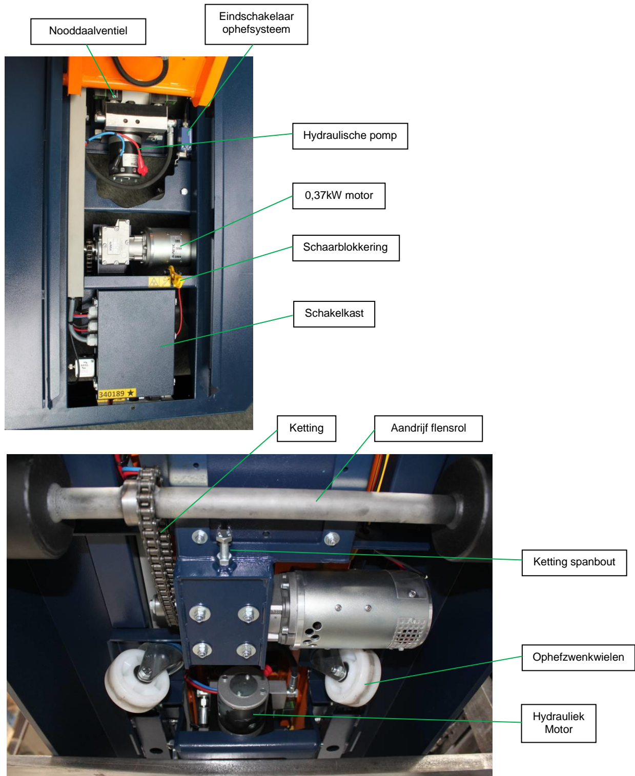
Figuur 5.2; Benaming van de onderdelen aan de onderzijde van de BENOMIC STAR
