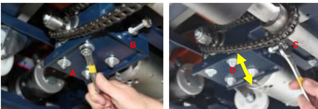
Figuur 9.5 A-B-C; Spannen van de ketting
