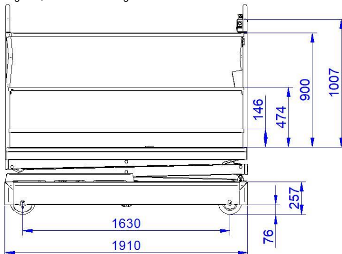
Fig. 2.5; Lengte afmetingen 2-schaar in mm
