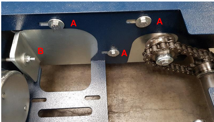
Figuur 9.5; Spannen van de ketting
