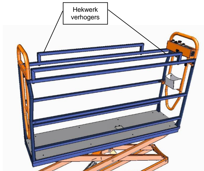
Figuur 5.1; Benaming van de onderdelen aan de bovenzijde van de BENOMIC S
