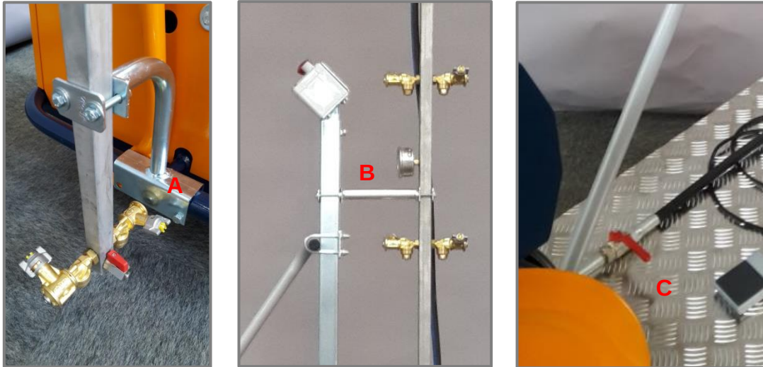
Figura 7.1: Installazione della lancia irroratrice
