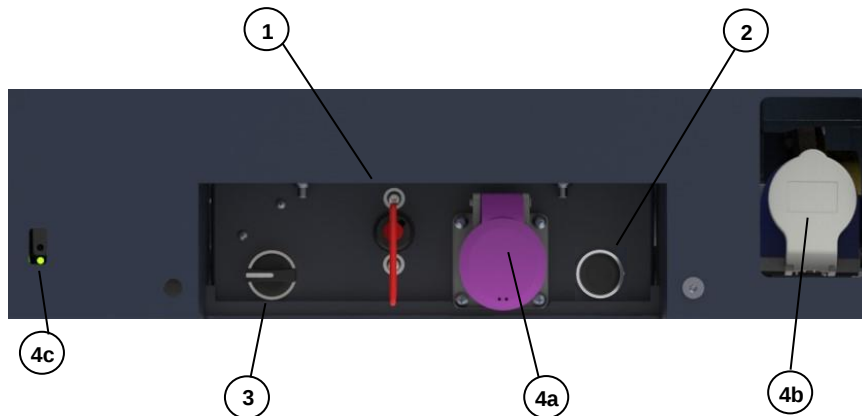
Figuur 8.1; Bediening op de onderwagen van de BeNomic Star PRO 350
