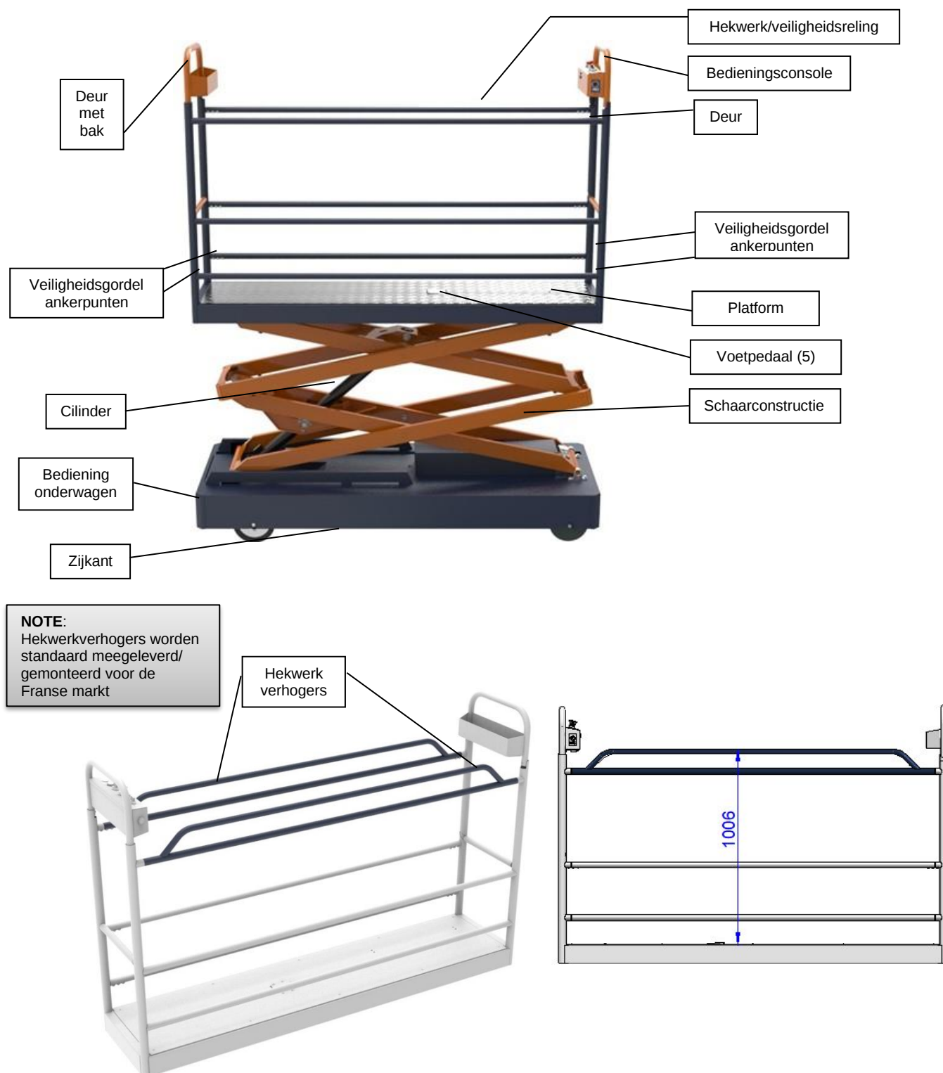
Figuur 5.1; Benaming van de onderdelen aan de bovenzijde van de BeNomic Star PRO 350
