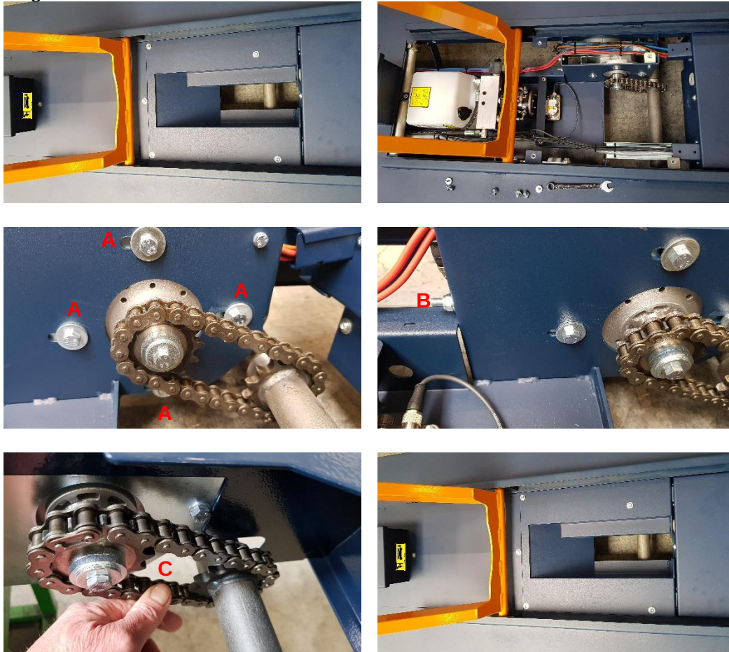
Figuur 9.3; Spannen van de ketting
