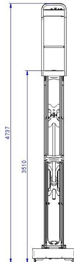
Fig. 2.2; Maximale hoogte afmetingen 2 schaar mm
