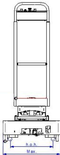
Fig. 2.1; Breedte afmetingen 2-schaar in mm
