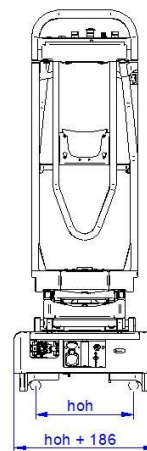
Fig. 2.1; Breedte afmetingen 2-schaar in mm
