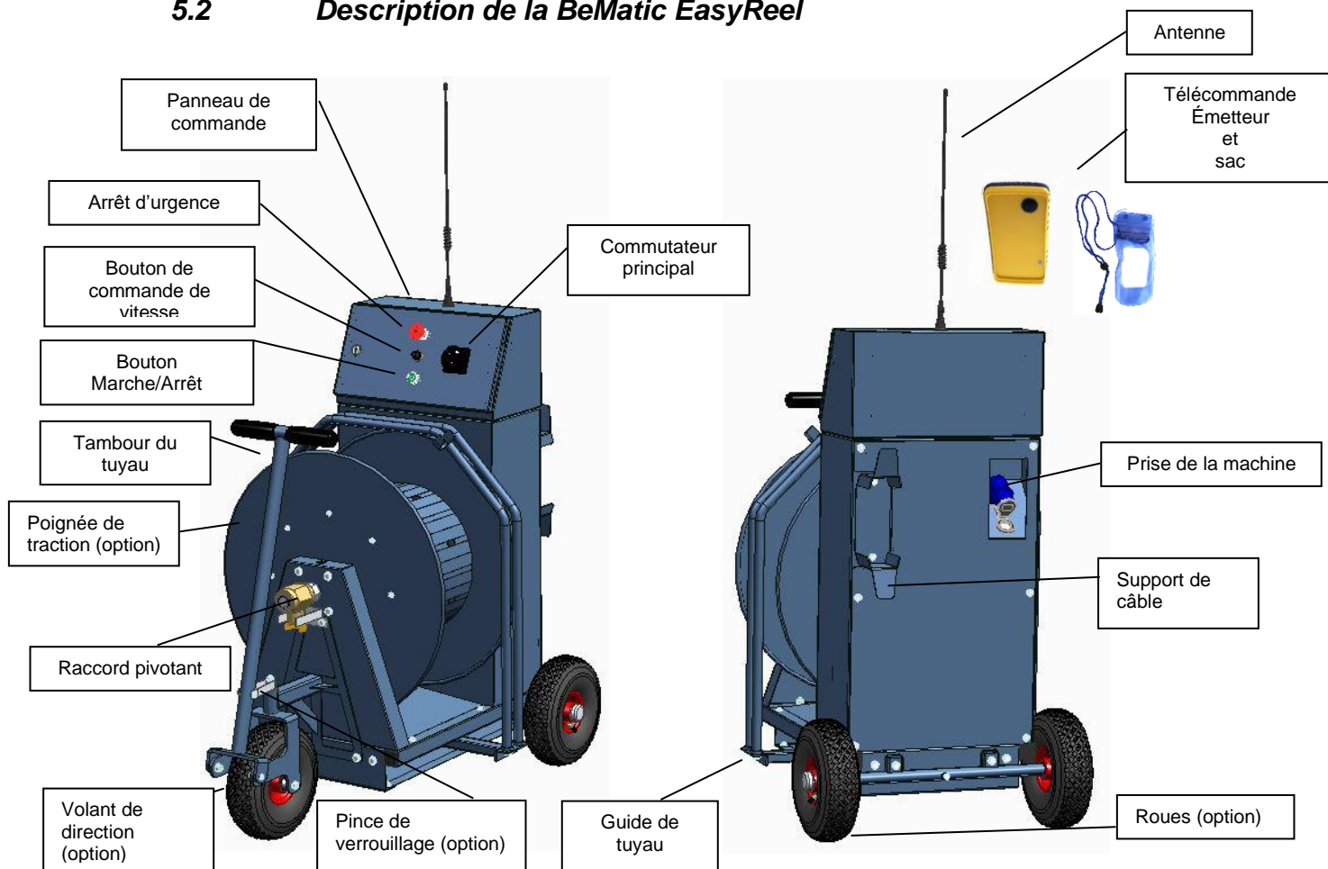
Figure 5.1 ; Noms des pièces de la BeMatic EasyReel
