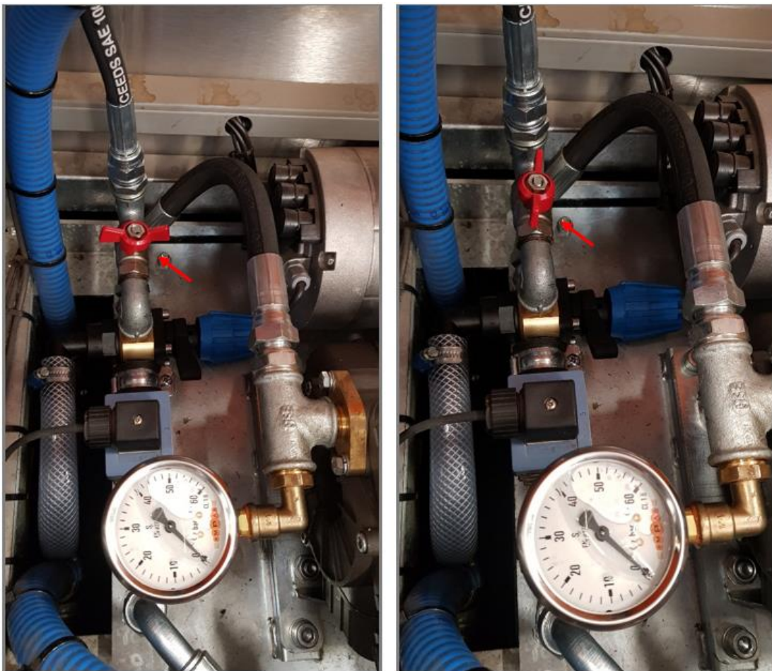
Ventil zavřený, míchací vstřikovač neaktivní
