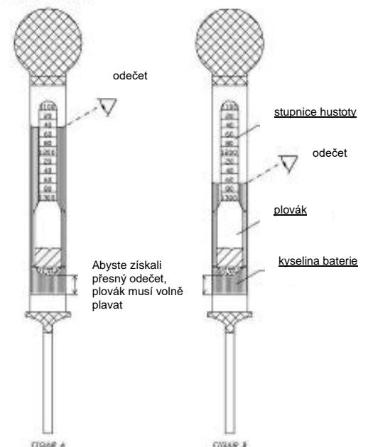
Nabitá baterie
